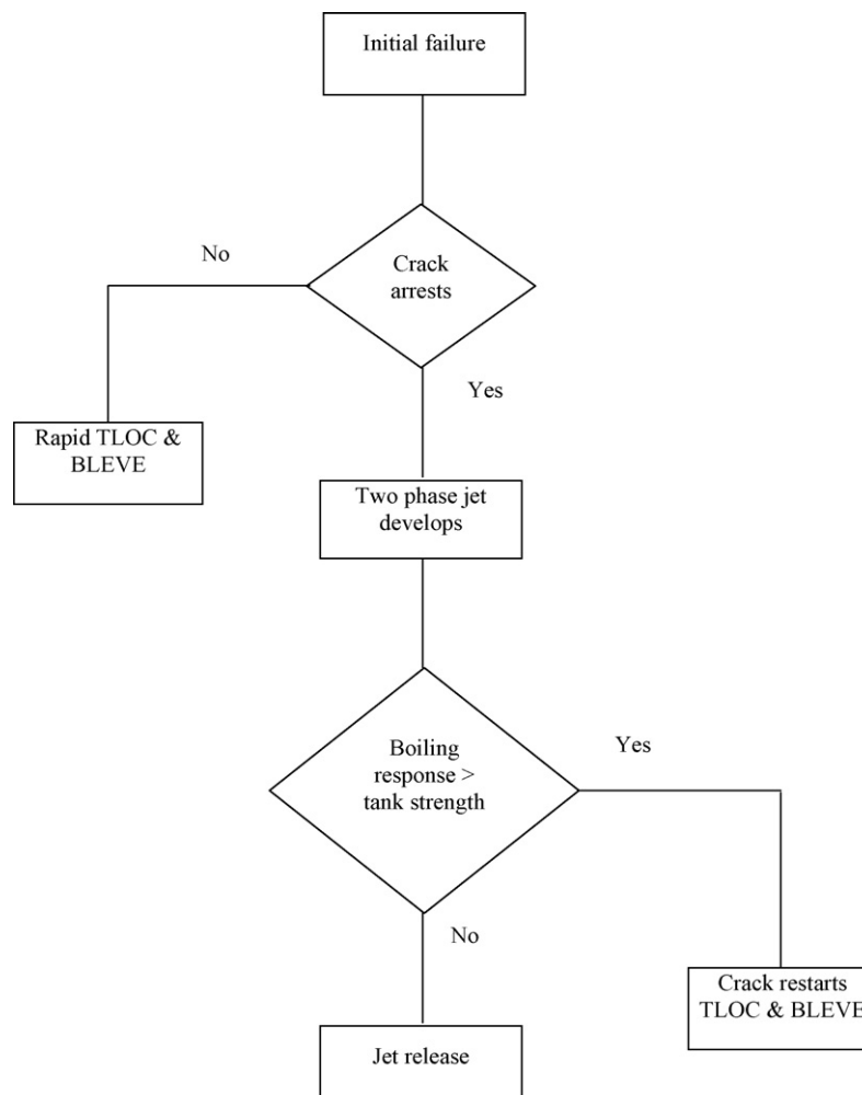
Fig. 2. Two-step BLEVE [2,64].
